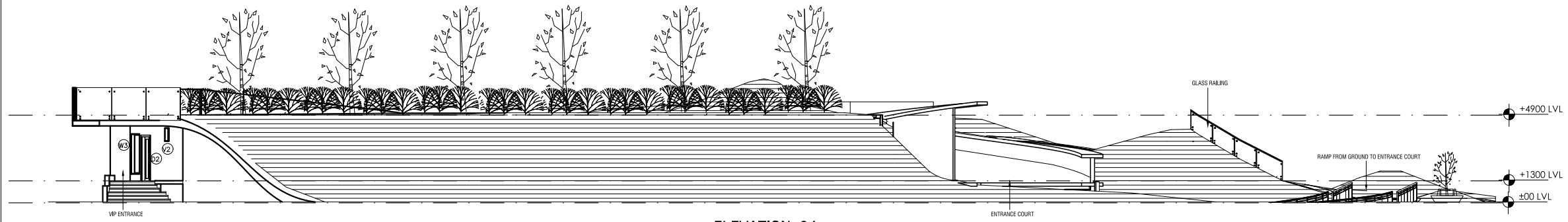
ELEVATION 04
